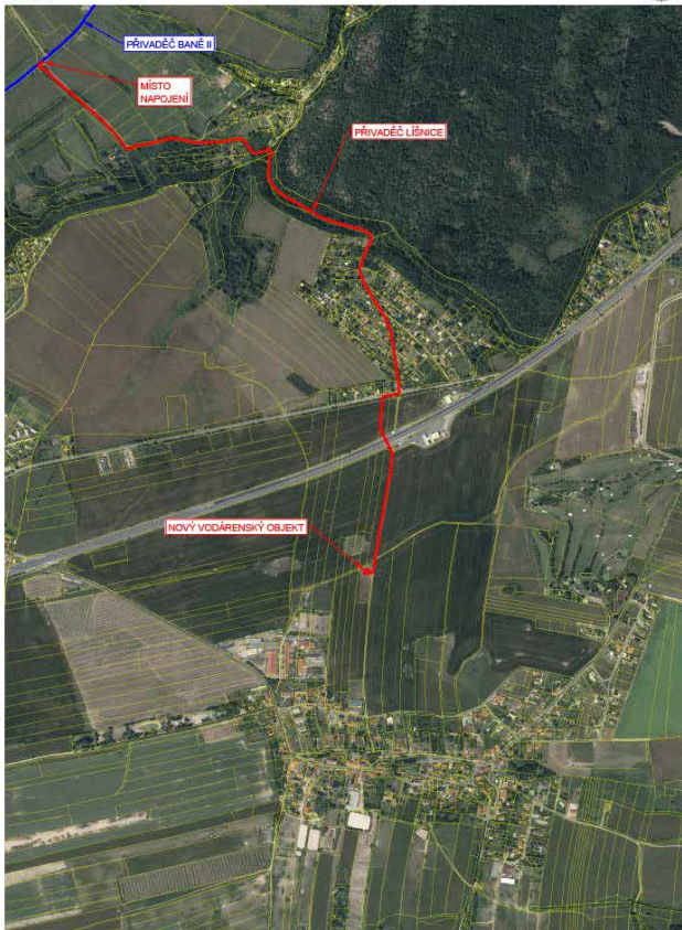
STUDIE NÁPOJENÍ OBCE LÍŠNICE NA VODOVODNÍ PŘIVADĚČ BANĚ II NÁVRH TRASY PRO PROJEDNÁNÍ 10/2025 M 1:10 000
